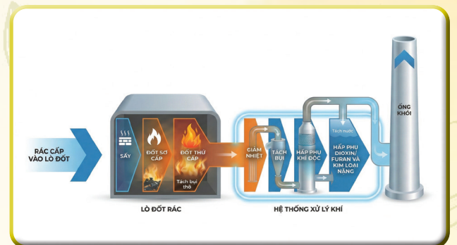
Sơ đồ cấu tạo thiết bị của lò đốt rác thải sinh hoạt T-TECH
