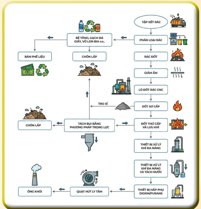
Sơ đồ công nghệ xử lý rác
