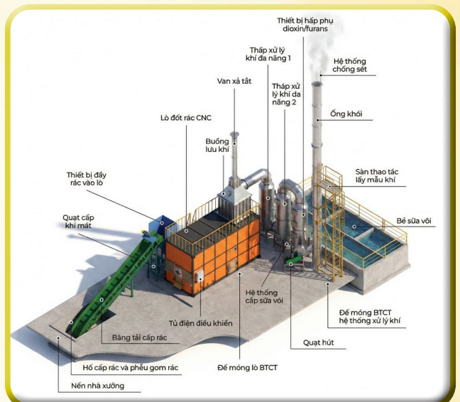
Nguyên lý hoạt động của lò đốt rác T-TECH
