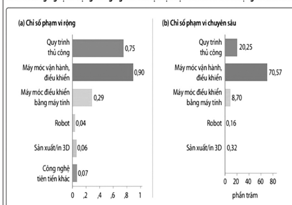
HÌNH 2: Công nghệ sử dụng trong ngành chế tạo tại Việt Nam theo chiều rộng và chiều sâu
